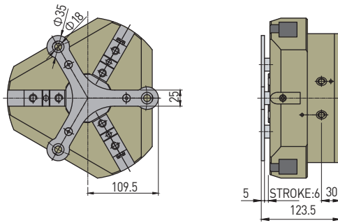
■ AF46SSA-160 DIMENSION
