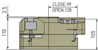
■ AF46SNA-160 DIMENSION
