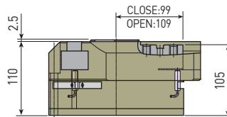
■ AF46SSA-160 DIMENSION
